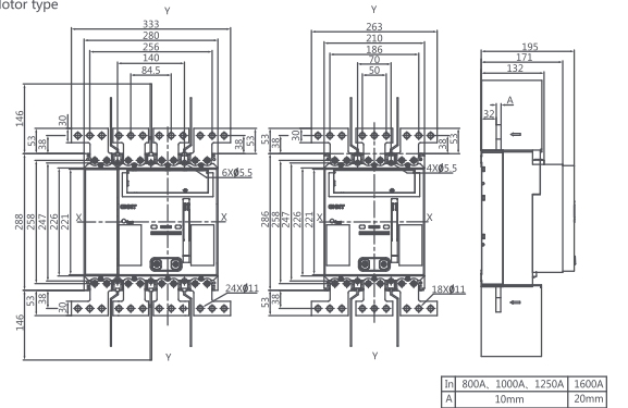
Diagram 5. NM8N(DC, SD)-1600
